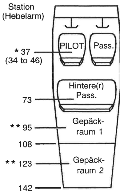
Abb. 6-3. Beladungsanordnung
