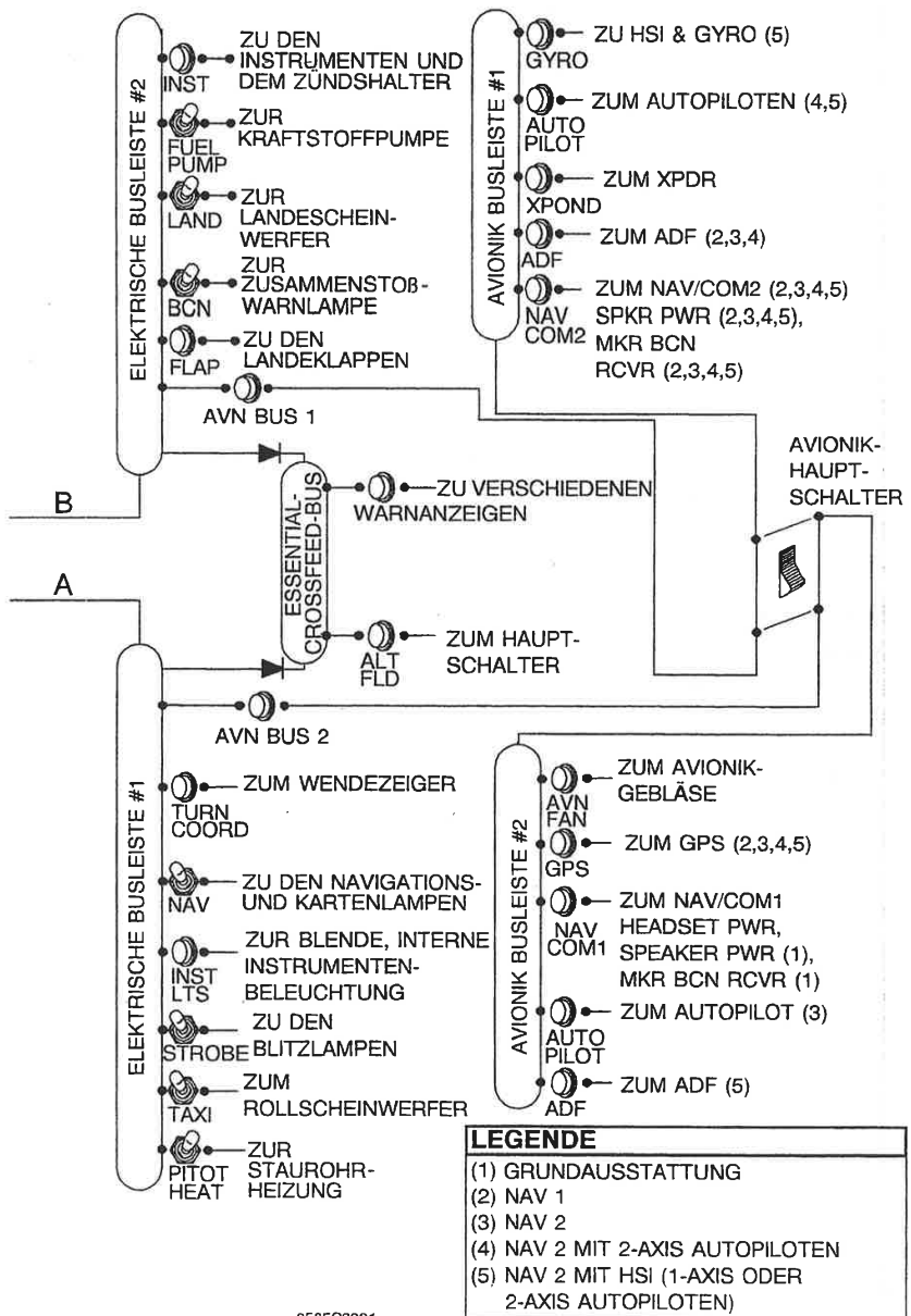
Abb. 7-7. Schema der elektrischen Anlage (Blatt 2 von 2)
