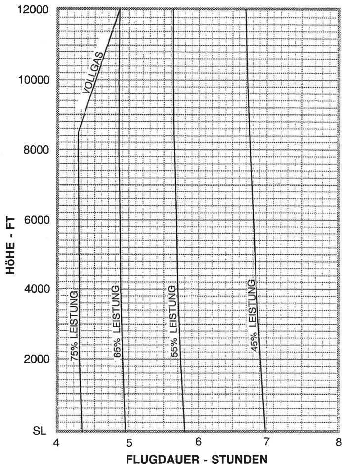
Abb. 5-10. Flugdauer
