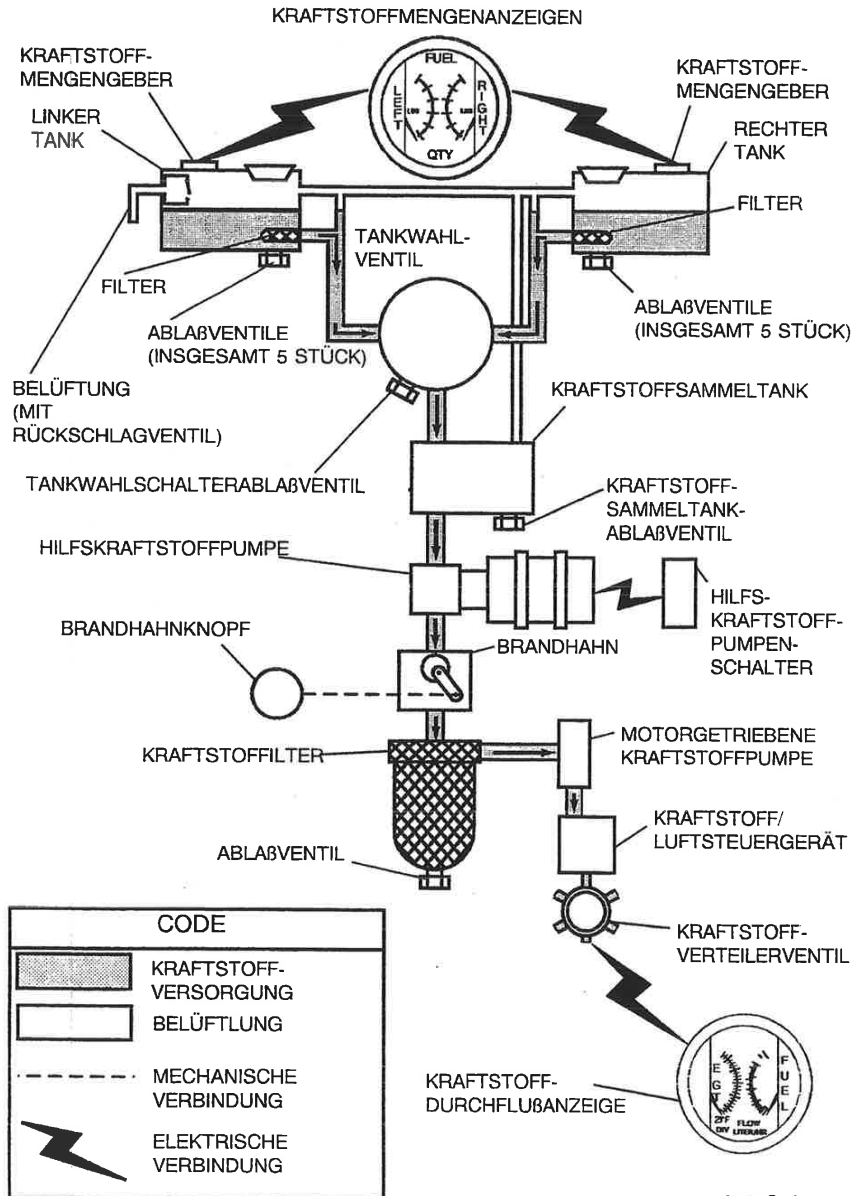
Abb. 7-6. Schema der Kraftstoffanlage
