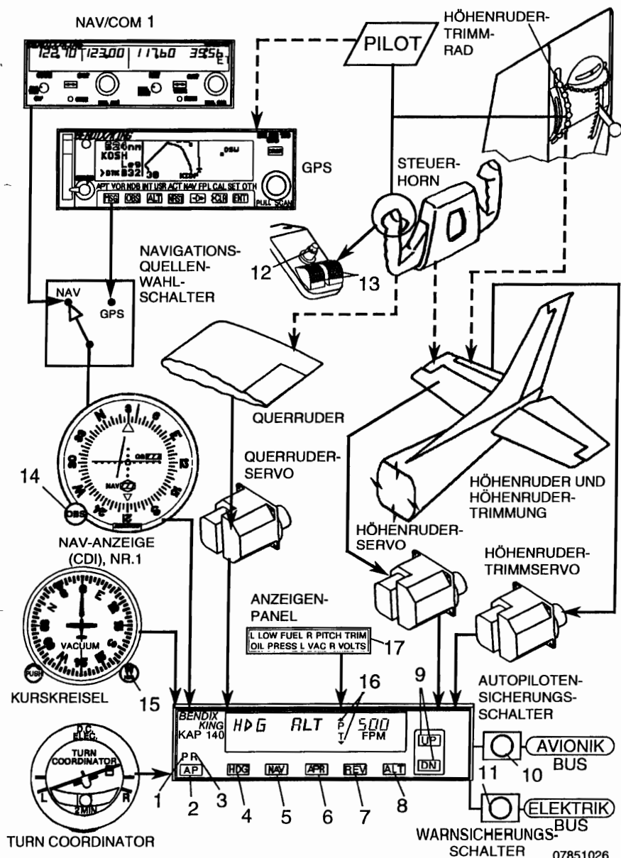
Abb. 1. Bendix/King KAP 140 2-Achs-Autopilot Bedienorgane und Anzeigen (Blatt 1 von 5)
