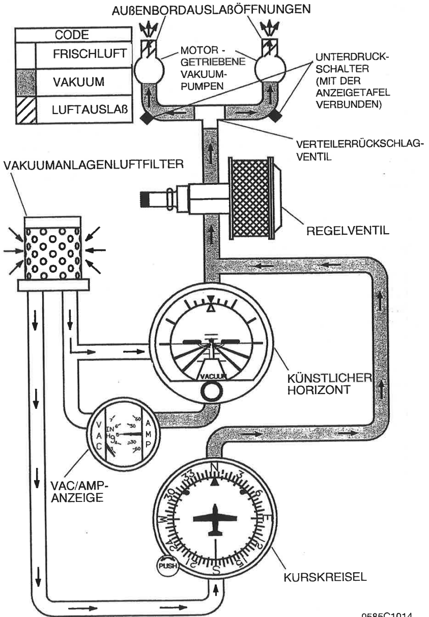
Abb. 7-9. Vakuumanlage
