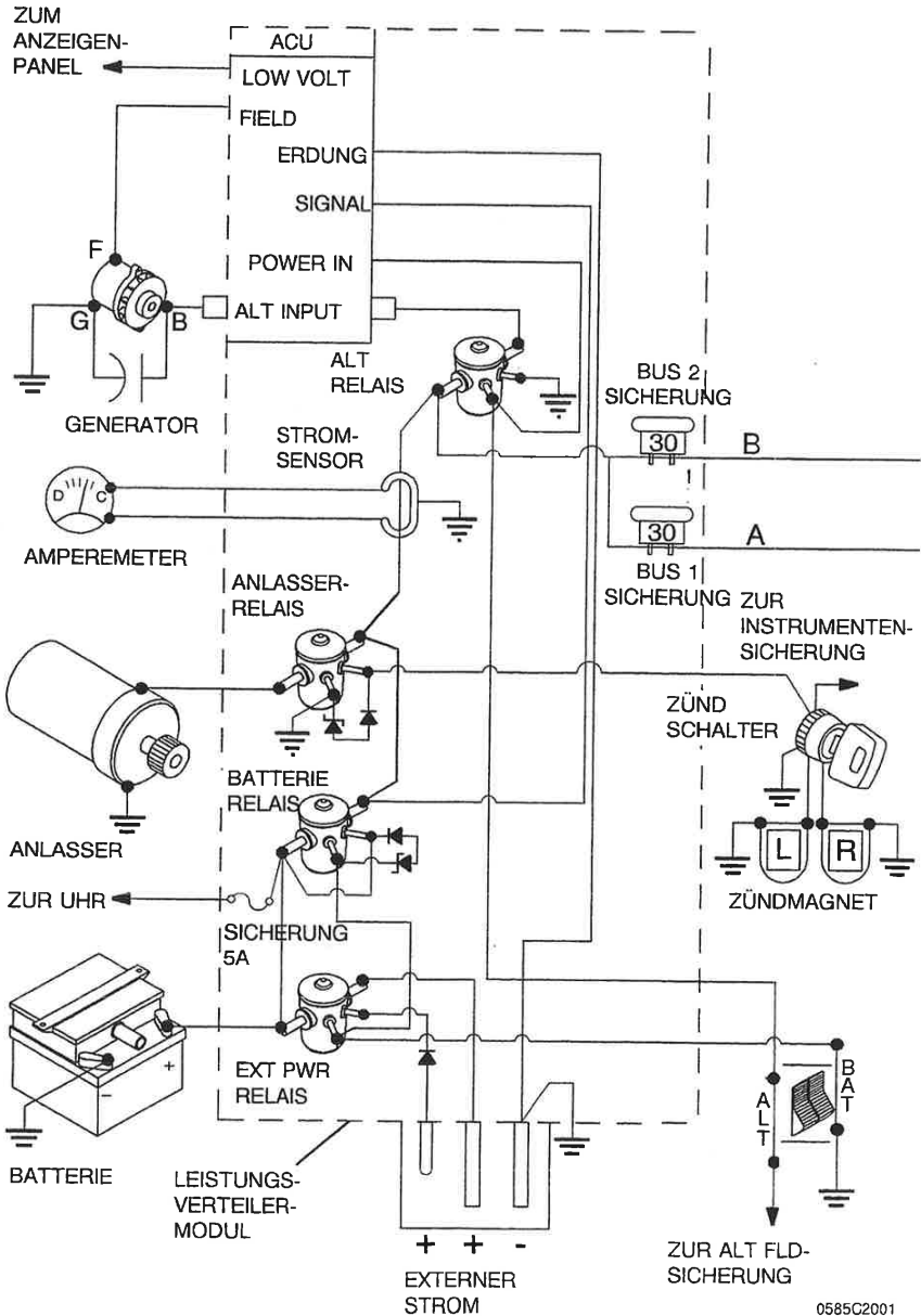
Abb. 7-7. Schema der elektrischen Anlage (Blatt 1 von 2)
