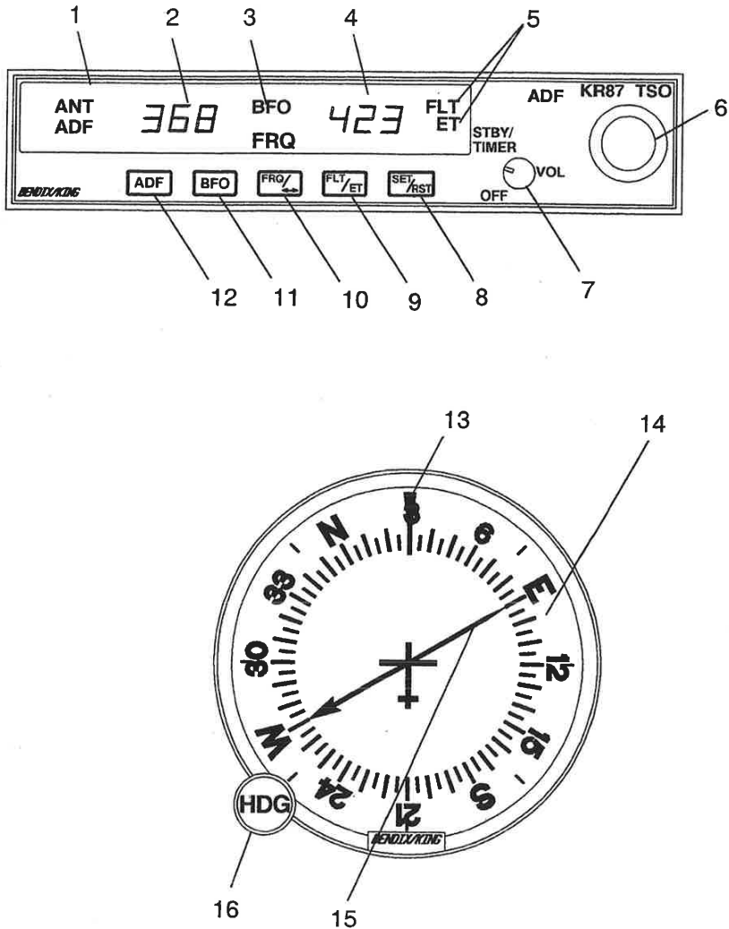
Abb. 1. KR 87 Radiokompaß (ADF) (Blatt 1 von 4)
