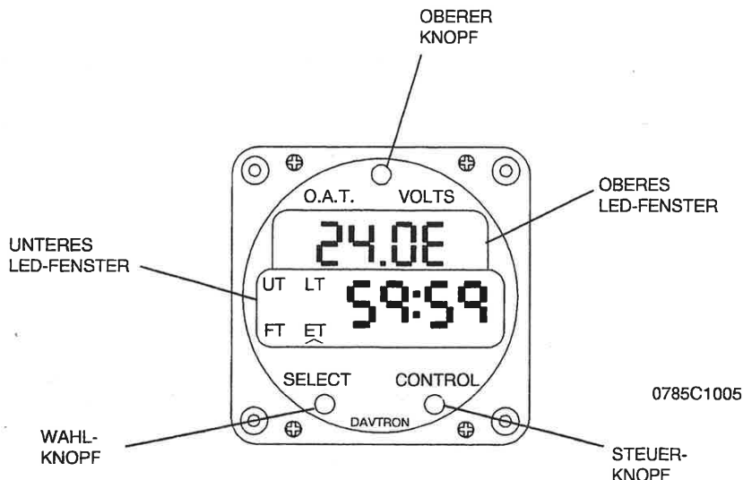
Abb. 1. Uhr / OAT-Anzeige
