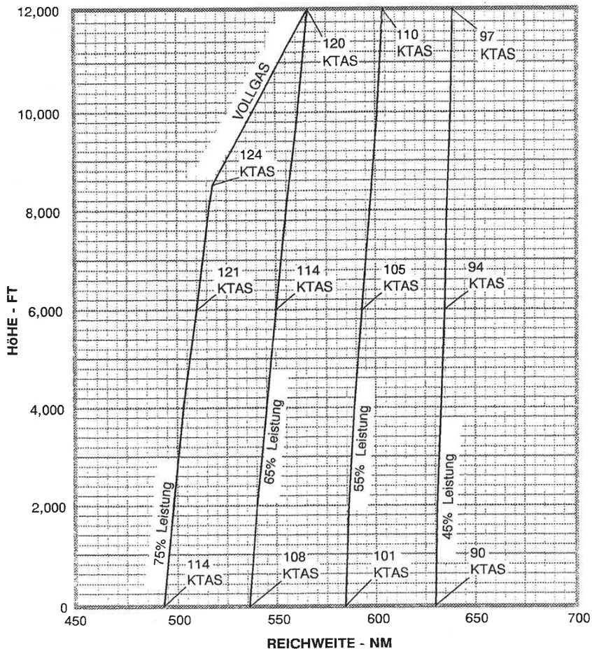
Abb. 5-9. Reichweite
