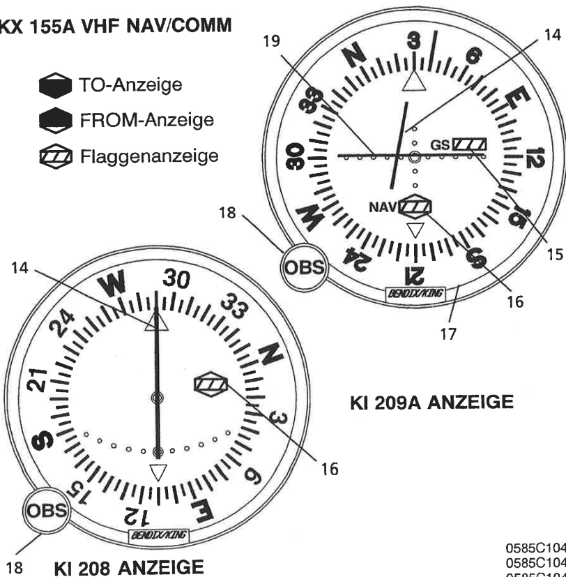
Abb. 1 Bendix/King KX 155A VHF NAV/COM mit KI 208 oder KI 209A Anzeige (Blatt 1 von 7)
