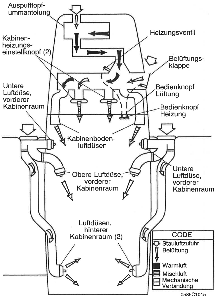
Figure 7-8. Kabinenheizungs-, Belüftungs- und Enteisungsanlage
